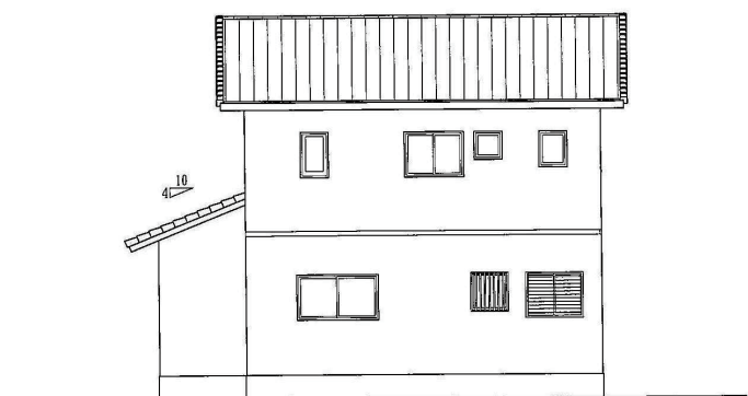
北側 立面図 S:1/100
