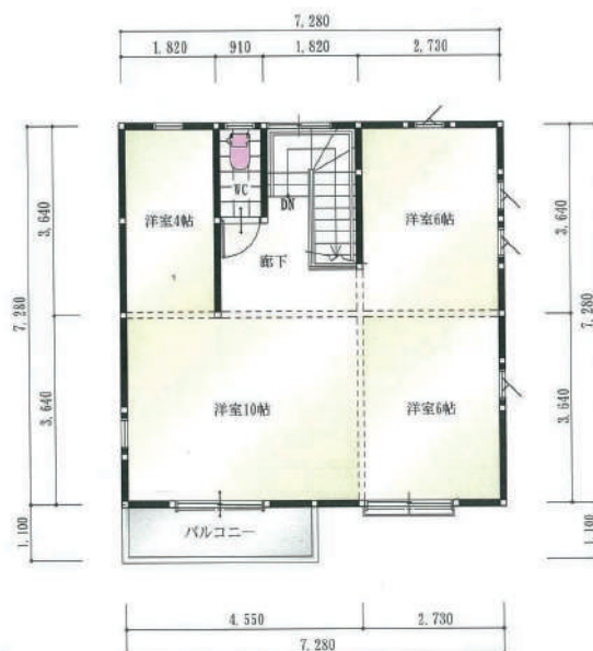
2階 平面図 S:1/100
